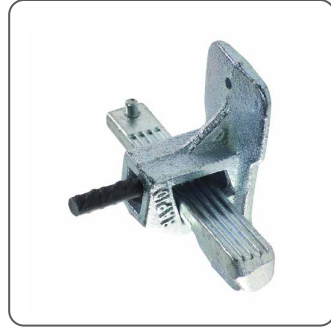
زرقينة بناء - إيطالي Rapid Clamp - Italy
